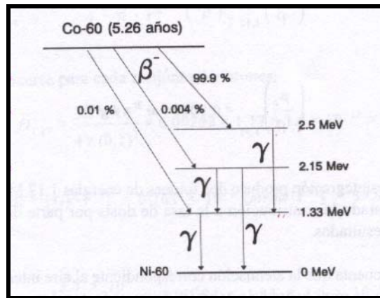
Figura 2: Esquema de desintegración del isótopo {}_{27}\text{Co}^{64} (4).
