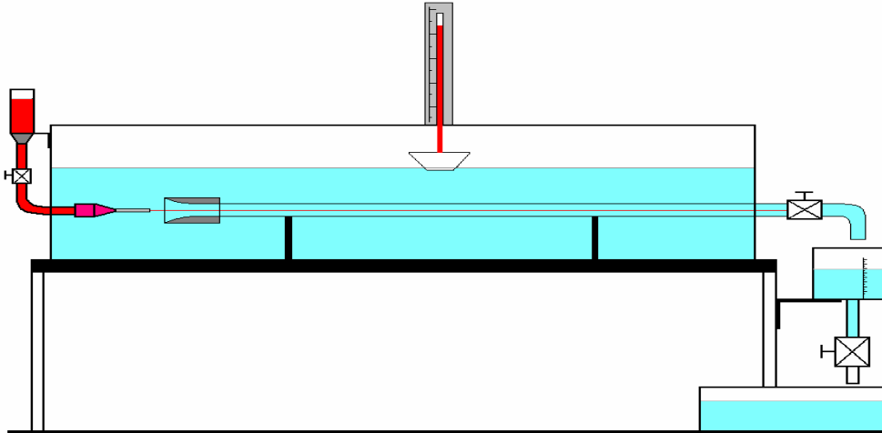
Figura 1. Dispositivo experimental propuesto para el experimento de Reynolds.
