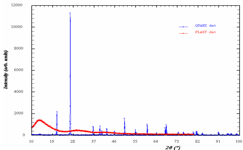
Figura 3. Espectros superpuestos del cuarzo (azul, con picos agudos) y un polímero amorfo (rojo, con halos en vez de picos).
